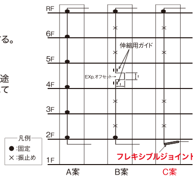
図4.2.1 立管の支持例
