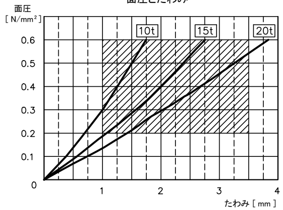
面圧とたわみ
