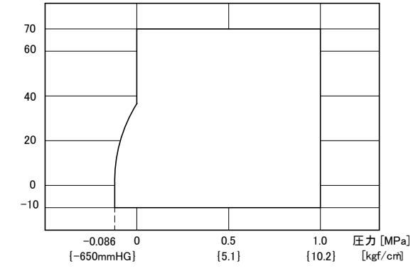
W-FLEX 使用範囲(温度・圧力)
